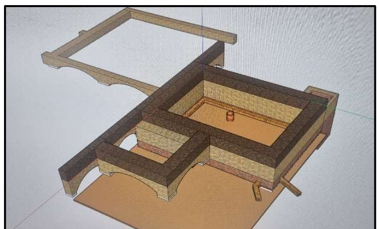
3D reconstructie van een deel van de fundatie zoals aangetroffen tijdens de recente opgraving en 1934. Deze fundering bevond zich geheel in de motte heuvel.
